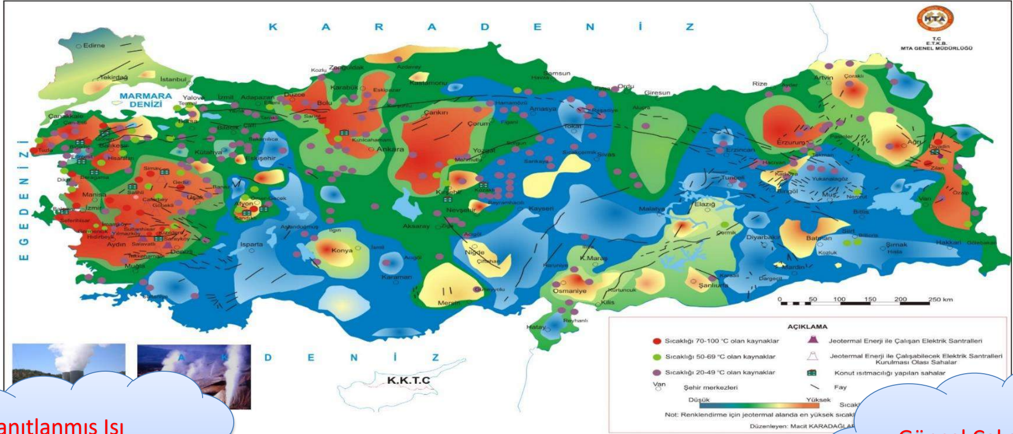
Jeotermal Kaynaklar ve Uygulama Haritası
